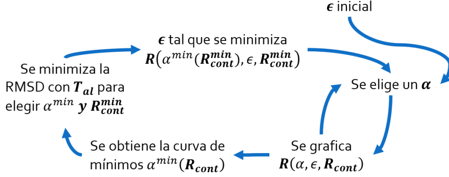
Figura 4.3: Esquema del algoritmo de optimización que se utilizó.
