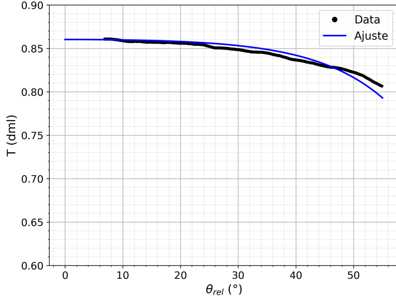
Figura 3.6: Transmitancia experimental y ajuste.
