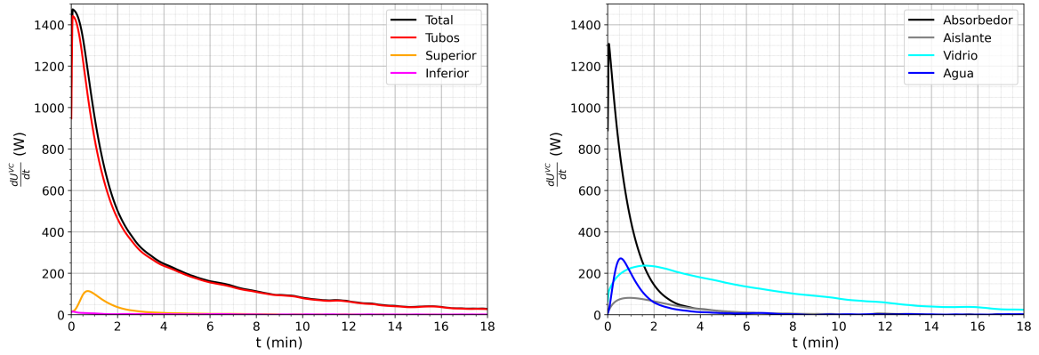
Figura 4.25: Energía almacenada en función del tiempo luego de retirarse la manta del colector. A la izquierda se distingue por sección y a la derecha por material.
