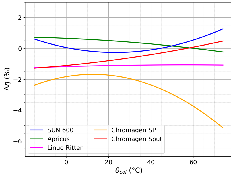
Figura 4.27: Diferencia entre rendimiento simulado y ensayado para los cinco modelos.
