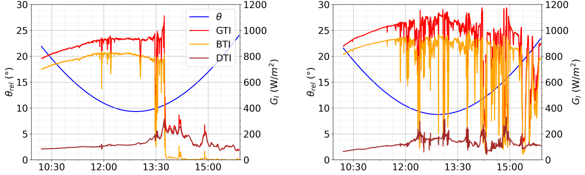
Figura 4.19: Irradiancias y ángulo de incidencia para el 3 de julio (izquierda) y el 9 de julio (derecha).
