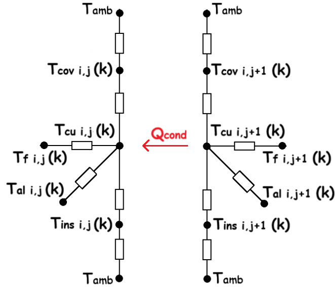
Figura 2.16: Diagrama de intercambios de calor entre volúmenes de control consecutivos. El índice k indica el paso temporal.
