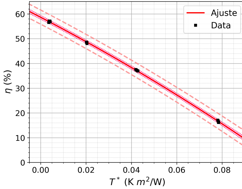
Figura 3.8: Medidas experimentales y ajuste del rendimiento contra la temperatura reducida.
