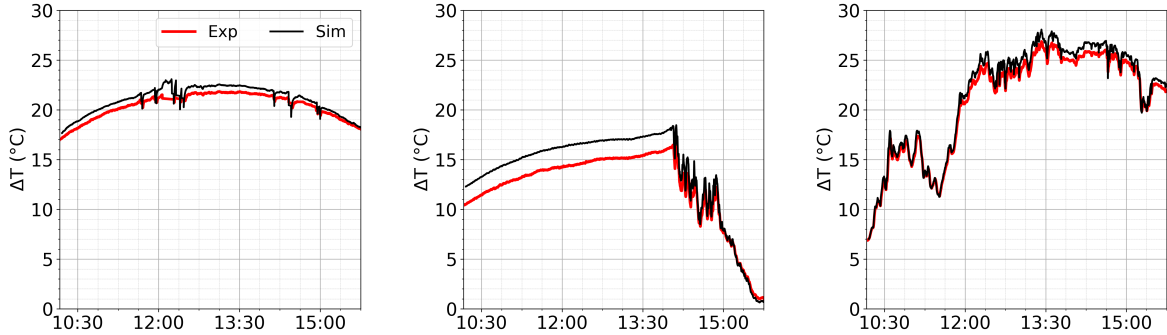
Figura 4.5: Para los tres días se muestra el promedio de la diferencia entre la temperatura de aluminio y de agua a la misma altura. Se contrastan resultados experimentales con simulaciones. Se fijaron los parámetros en \alpha = 0.88 , \epsilon = 0.33 y R_{\text{cont}} = 19 \times 10^{-4} \text{ Km}^2/\text{W} .
