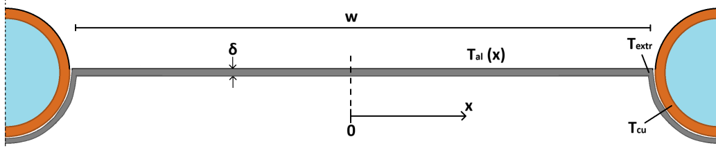
Figura 2.5: Esquema del análisis térmico en las aletas.
