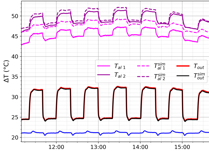
Figura 4.16: Comparación de los cambios de temperatura en el agua de salida al variar el caudal.
