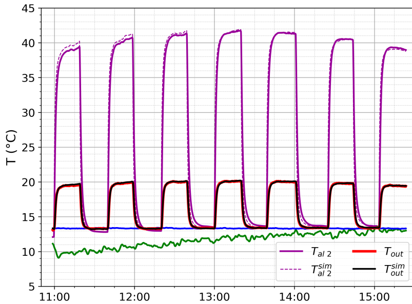
Figura 4.13: Comparación entre las curvas de temperatura de salida y de aluminio en función del tiempo.
