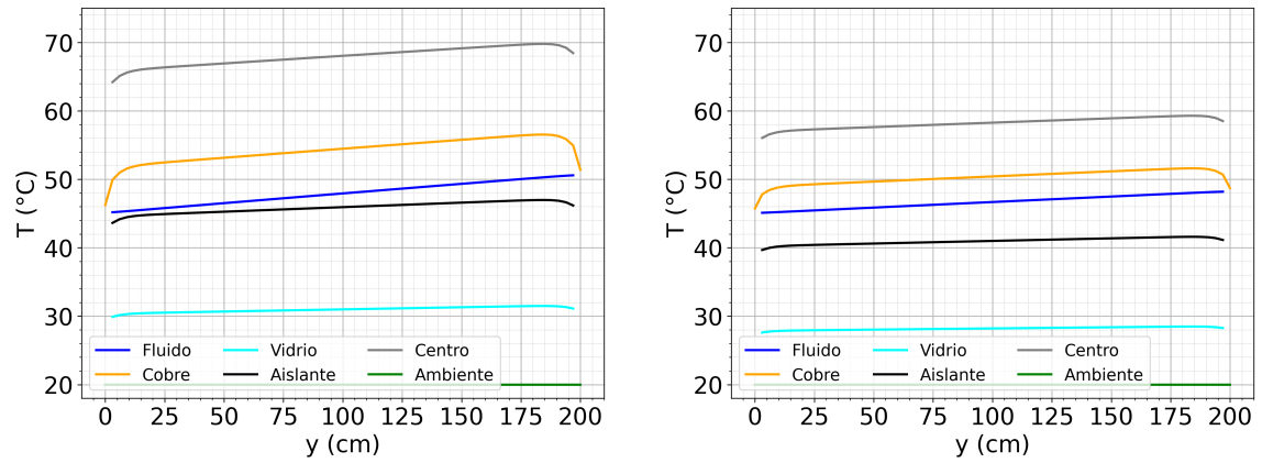
Figura 2.19: Se muestra el perfil de temperaturas en la dirección axial en el colector, a la izquierda para un día de cielo claro y a la derecha para un día parcialmente nublado.
