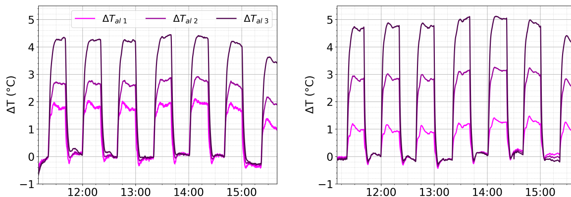
Figura 4.17: Saltos de temperatura en el aluminio entre la temperatura con caudal máximo (0 °C) y con mínimo para las tres termorresistencias. A la izquierda se encuentran las medidas y a la derecha las simulaciones.
