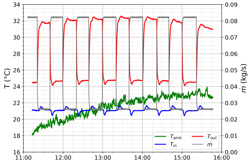
Figura 3.14: Temperaturas y caudal en función del tiempo.
