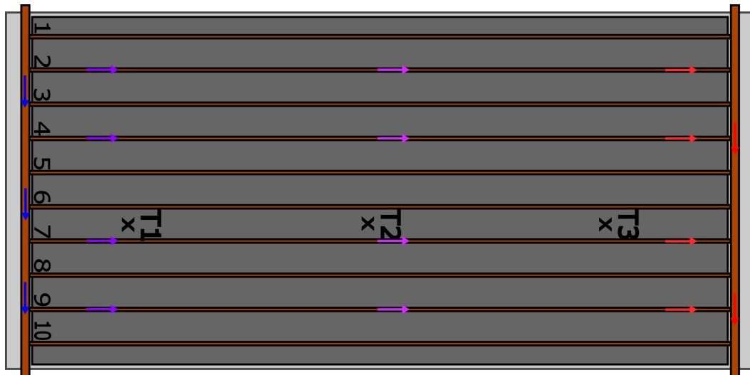
Figura 3.1: Esquema de la placa absorbedora y los tubos de cobre por los que circula agua.
