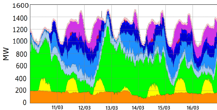
Figura 1.3: Consumo eléctrico del país estimado por ADME entre el 10 y el 17 de marzo. Extraído de su página web el 24 de marzo de 2025. Los colores indican la fuente energética utilizada: biomasa (anaranjado), solar (amarillo), eólica (verde), hidráulica (azules), roja (térmica) e importaciones.
