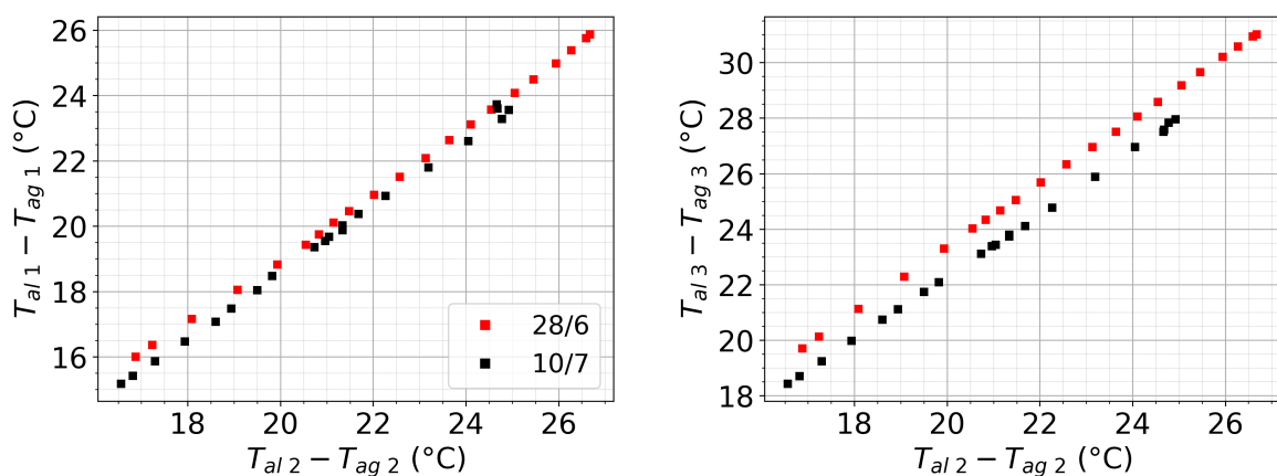
Figura 3.18: En el panel izquierdo se muestran la diferencia de temperaturas entre el aluminio y el agua dentro del tubo para la altura más baja contra la del medio. A la derecha se observa la misma diferencia para la termorresistencia más alta contra la segunda.
