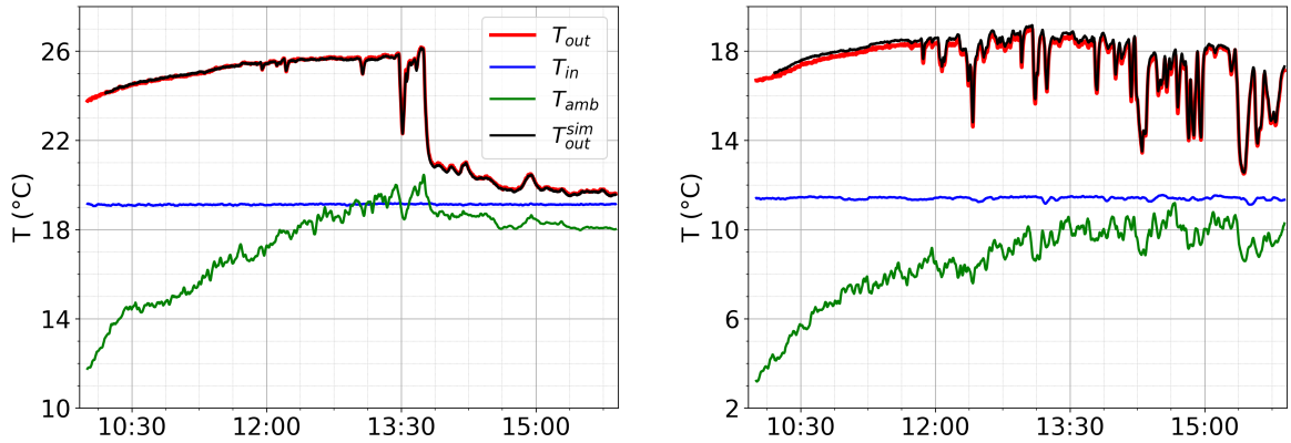
Figura 4.20: Temperaturas de entrada, salida y ambiente para el 3 de julio (izquierda) y el 9 de julio (derecha).
