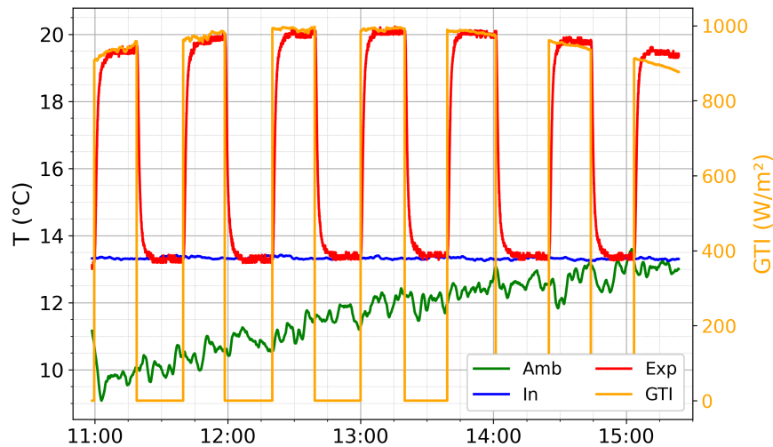
Figura 3.12: Temperatura e irradiancia en función del tiempo al momento de retirar la manta del colector.
