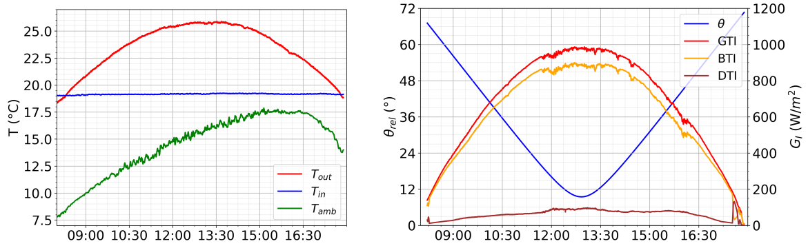
Figura 3.10: En el panel de la izquierda se muestran las temperaturas en función del tiempo y a la derecha se muestra la irradiancia y el ángulo incidente.
