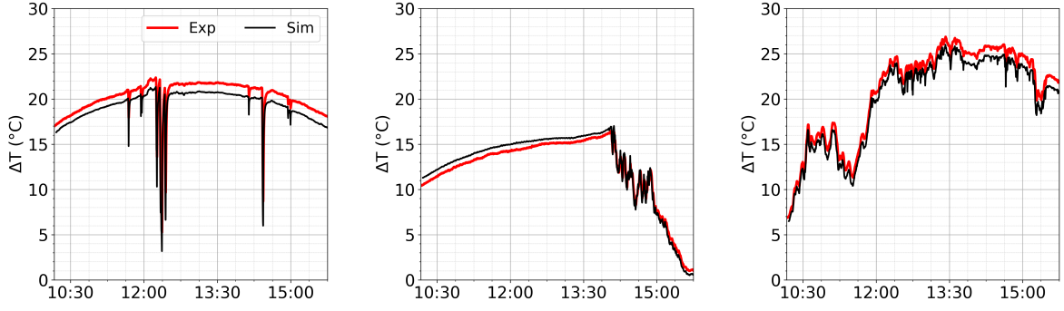
Figura 4.6: Para los tres días se muestra el promedio de la diferencia entre la temperatura de aluminio y de agua a la misma altura. Se contrastan resultados experimentales con simulaciones. Se fijaron los parámetros en \alpha = 0.87 , \epsilon = 0.33 y R_{\text{cont}} = 13 \times 10^{-4} \text{ Km}^2/\text{W} .
