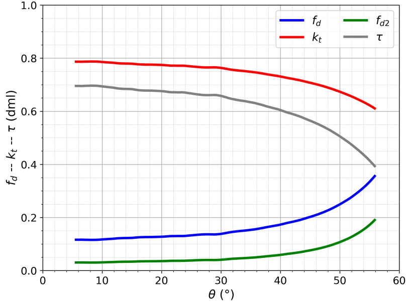
Figura 3.4: Fracciones difusas definidas, índice de claridad y transmisividad de la atmósfera.
