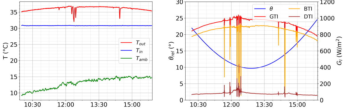
Figura 3.7: En el panel de la izquierda se muestran las temperaturas en función del tiempo y a la derecha se muestra la irradiancia incidente.
