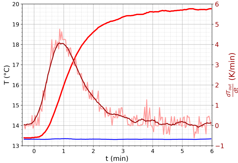
Figura 3.13: Temperatura y su derivada para los minutos siguientes al retirar la manta del colector.
