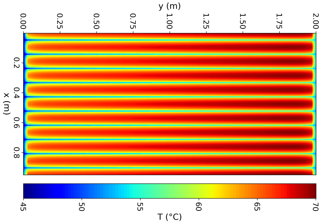
Figura 2.17: Temperatura del absorbedor para el estado estacionario con el agua ingresando a 45 °C en condiciones de cielo claro.
