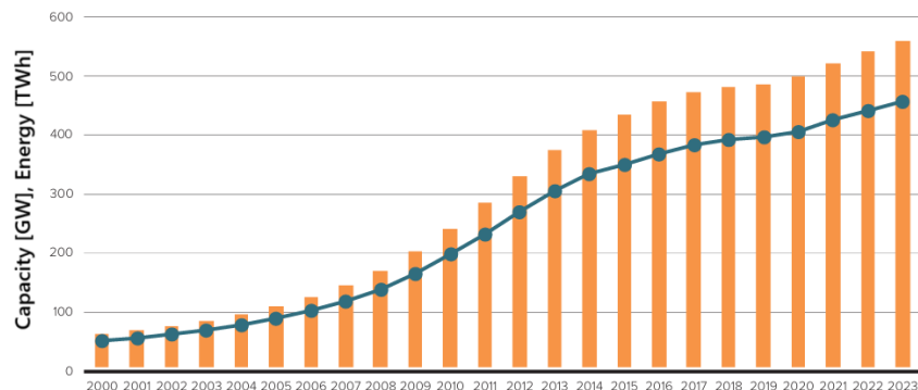
Figura 1.4: Se muestra la potencia instalada y energía producida por año desde el 2000 al 2023. Extraída del Informe de Weiss y Spörk-Dür, 2023.
