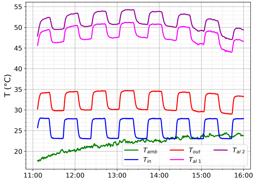
Figura 3.16: Ascenso y descenso de las temperaturas medidas al variar T_{\text{ing}} como función del tiempo.
