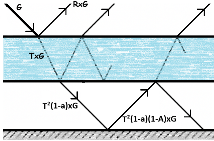
Figura 2.14: Esquema sobre cómo se dan las reflexiones y las transmisiones en el sistema. G es la irradiación solar, T y T' son las transmisividades aire-vidrio y viceversa, R es la reflectividad y A es la absorptividad de la pintura.
