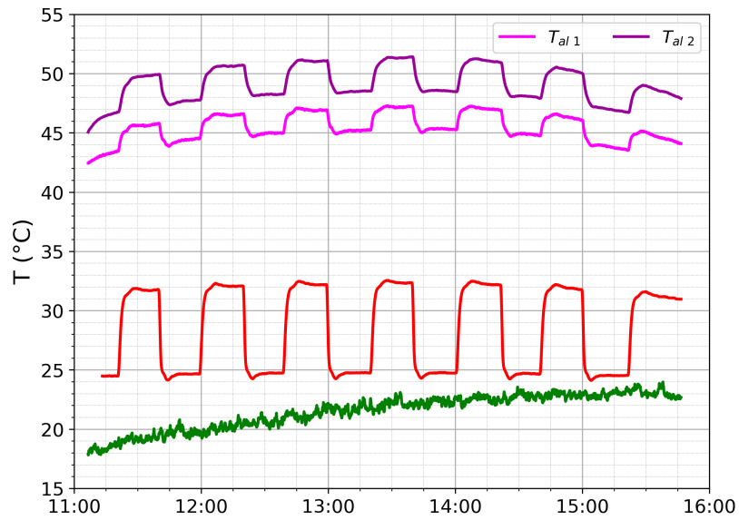
Figura 3.15: Ascenso y descenso de las temperaturas medidas en el aluminio al variar \dot{m} como función del tiempo.
