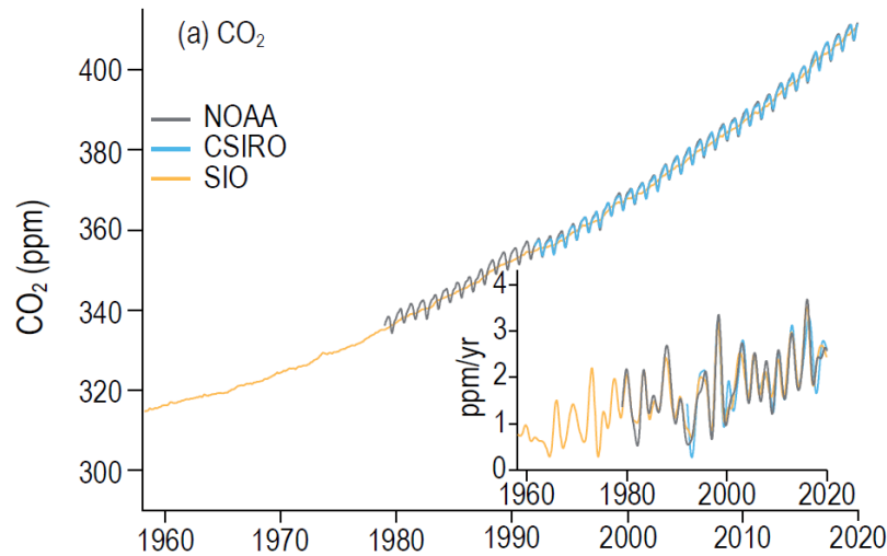
Figura 1.2: Concentración del dióxido de carbono a lo largo de los años medida en el laboratorio Mauna Loa de la NOAA. Se observa también su derivada. Extraída de Masson-Delmotte et al. 2021
