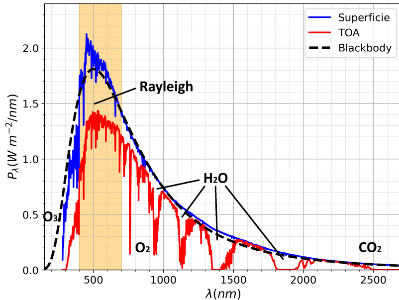
Figura 1.1: Espectro de la radiación solar en el TOA.
