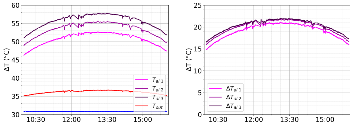
Figura 4.1: En el panel de la izquierda se muestran las temperaturas en función del tiempo medidas y a la derecha se muestra la diferencia de entre el aluminio y el agua a la misma altura del tubo ascendente.
