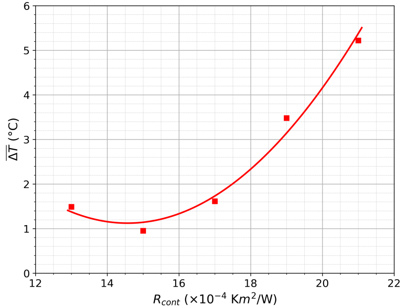
Figura 4.7: Diferencia cuadrática media entre \Delta T de la simulación y las medidas del 28 de junio.
