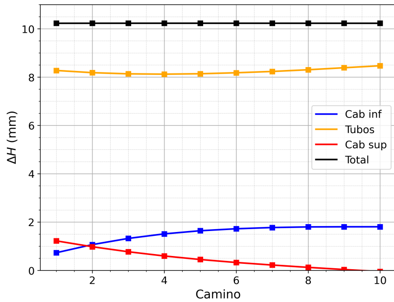
Figura 2.12: Pérdidas de carga estimadas en función del camino.
