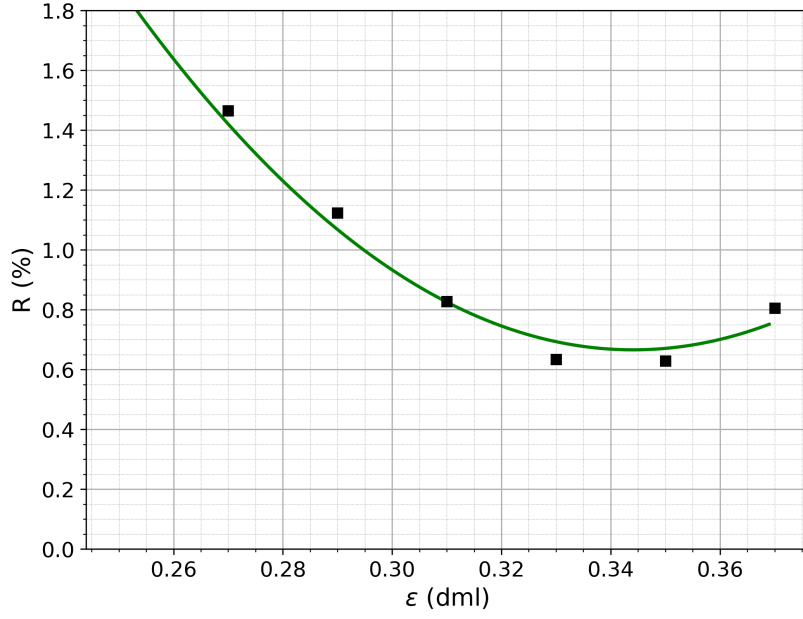
Figura 4.8: Diferencia cuadrática media entre \eta(T^*) de la simulación y las medidas con los valores óptimos de \alpha y R_{\text{cont}} variando la emisividad.
