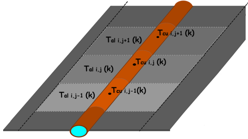
Figura 2.15: Esquema que muestra algunos volúmenes de control de cobre y de aluminio.
