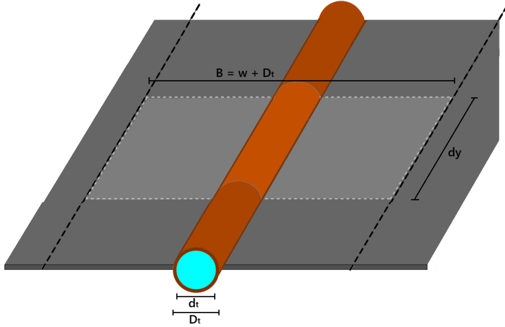
Figura 2.4: Visualización del volumen de control de aluminio y de cobre.
