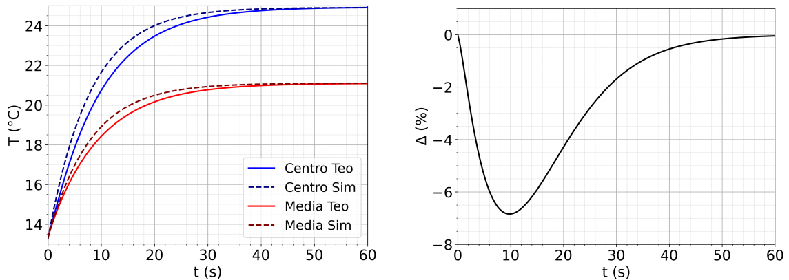
Figura 2.8: A la izquierda se muestra el ascenso de la temperatura media del aluminio y de la temperatura en el extremo adiabático de la aleta. Del lado derecho se muestra el error porcentual para la simulación y el caso teórico.
