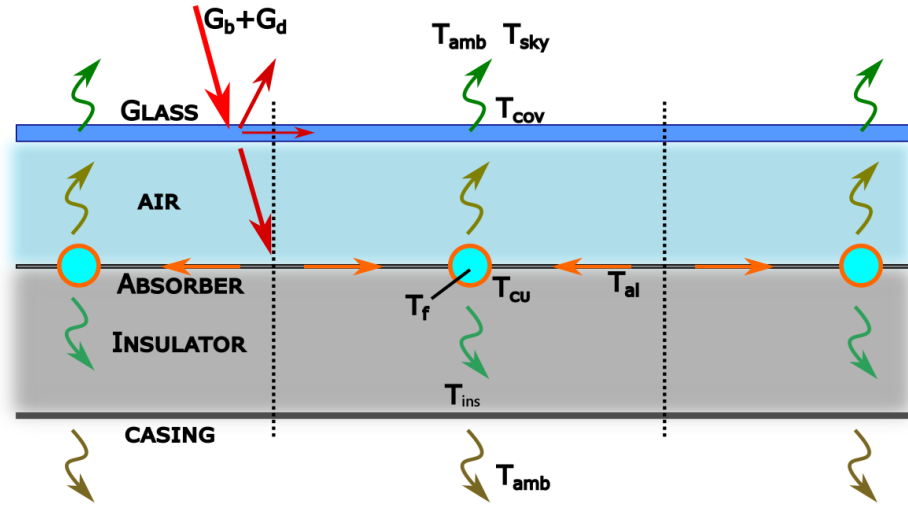
Figura 2.2: Corte esquemático al FPSC donde se visualiza la estructura en la dimensión menor.
