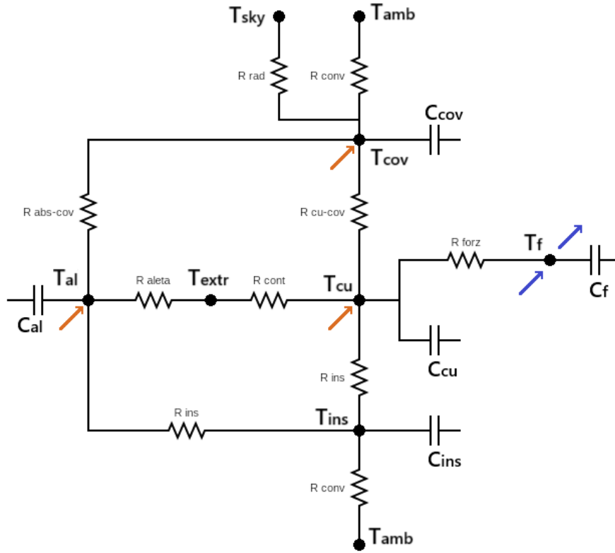
Figura 2.3: Diagrama de resistencias y capacitancias térmicas del colector solar. Con flechas naranjas se indican los ingresos de calor solar y en azul el calor de transporte del flujo.
