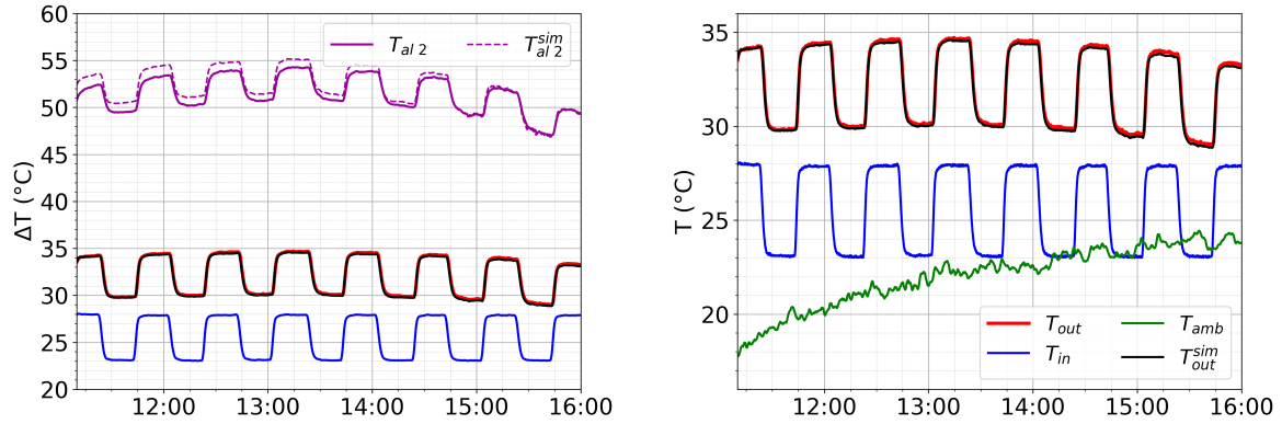
Figura 4.18: Saltos de temperatura en el aluminio entre la temperatura con caudal máximo (0 °C) y con mínimo para las tres termorresistencias.
