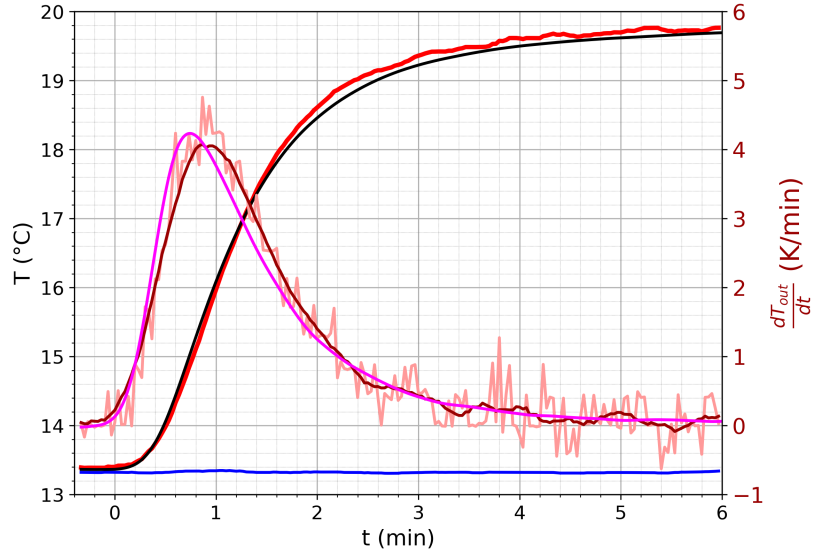
Figura 4.14: Comparación de la temperatura del agua de salida y su derivada para una sola subida.
