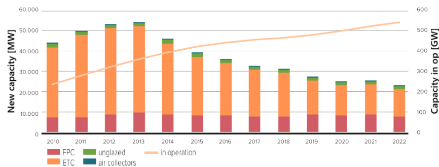
Figura 1.6: Nueva potencia instalada y nueva energía producida año a año discriminada por el tipo de energía. Extraída del Informe Weiss y Spörk-Dür, 2023.
