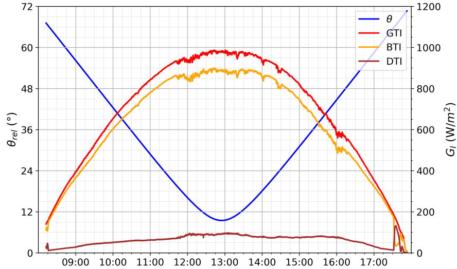
Figura 4.10: Medidas de irradiancia e incidencia angular durante el ensayo de IAM.
