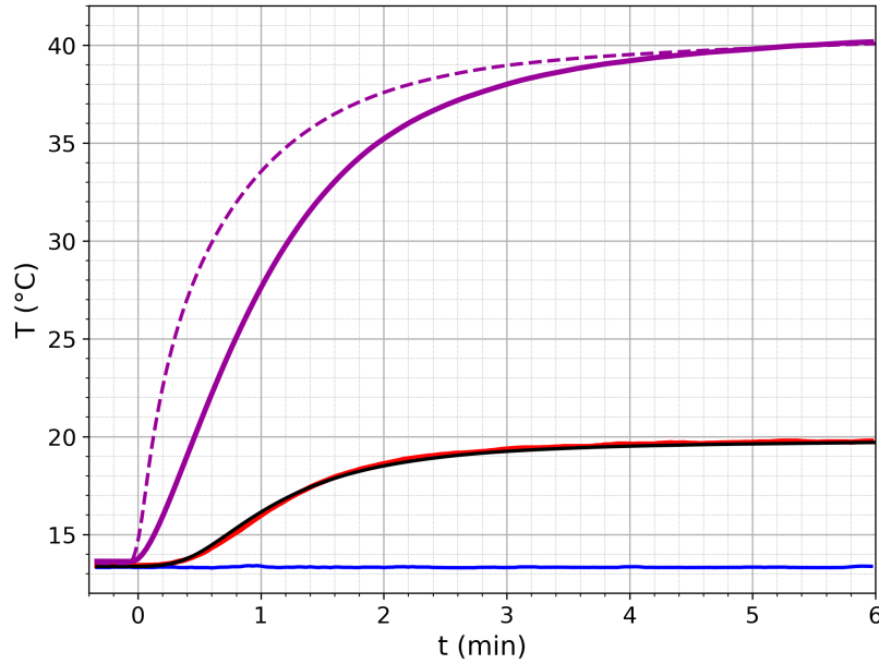
Figura 4.15: Comparación de la suba de temperatura del aluminio. Se observa una demora en la subida experimental.
