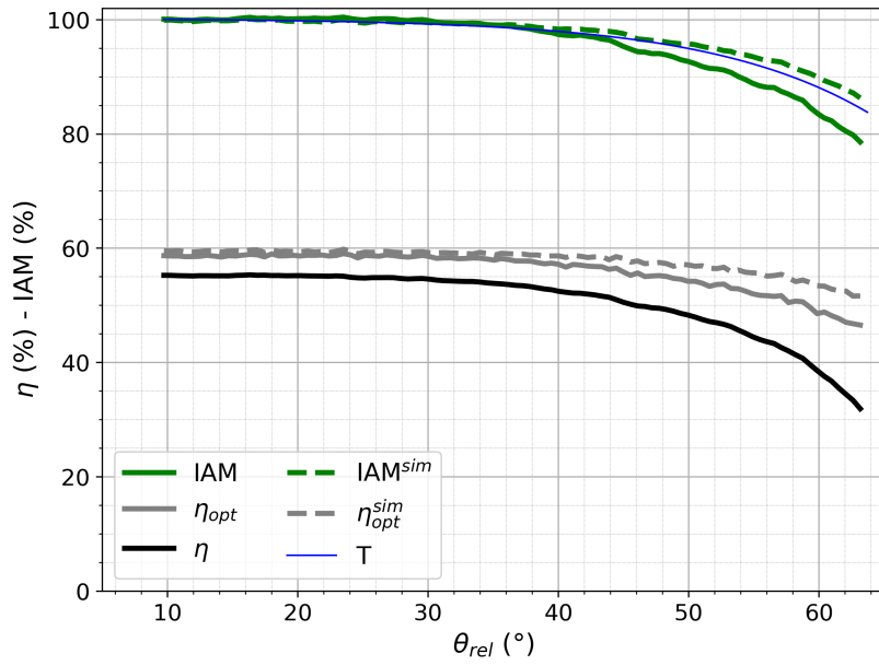
Figura 4.12: Curvas de rendimiento y IAM en función del ángulo de incidencia.
