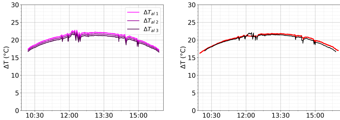
Figura 4.2: En el panel de la izquierda se muestran las temperaturas en función del tiempo simuladas con R_{\text{cont}}=15 \times 10^{-4} \text{ Km}^2/\text{W} y a la derecha se muestra la diferencia de entre aluminio y agua en promedio comparando experimental y simulada.
