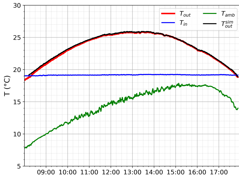
Figura 4.11: Medidas de temperatura ambiente, entrada y salida durante el ensayo de IAM.
