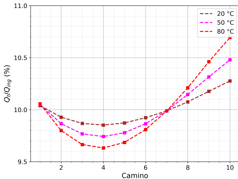
Figura 2.13: Distribución de caudal en función del camino.
