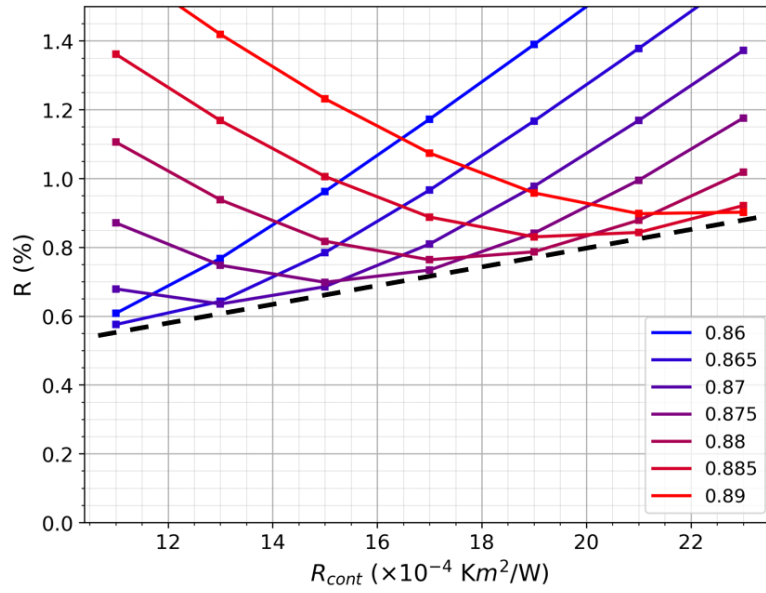
Figura 4.4: Valor de R promedio para las curvas \eta(T^*) para varios juegos de parámetros. Se fijó el valor de \epsilon en 0.33, la leyenda indica el valor de \alpha .
