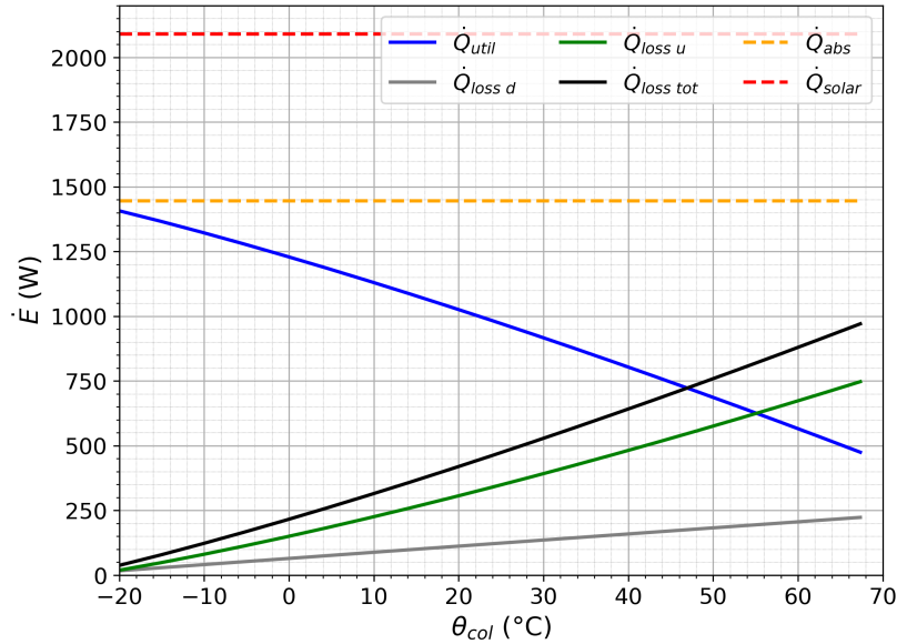
Figura 4.22: Pérdidas y calor útil del colector en condiciones nominales.
