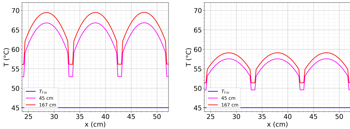
Figura 2.18: Se muestra el perfil de temperaturas para dos tubos del colector, a la izquierda para un día de cielo claro y a la derecha para un día parcialmente nublado.
