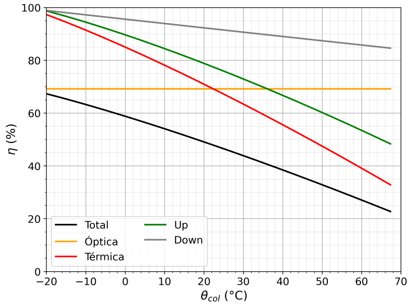
Figura 4.23: Rendimientos del colector en condiciones nominales.
