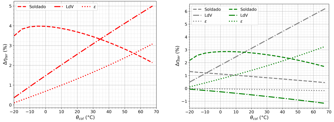
Figura 4.24: Aumento de rendimiento térmico con respecto a Baroni (izquierda) y su descomposición el rendimiento por arriba y por abajo (derecha).
