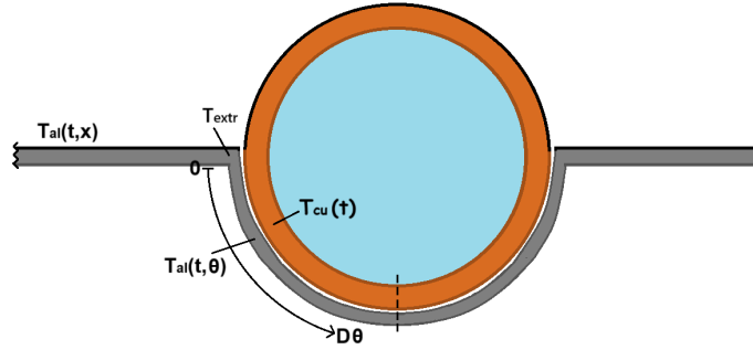
Figura 2.9: Esquema del modelado de la resistencia de contacto como aleta.
