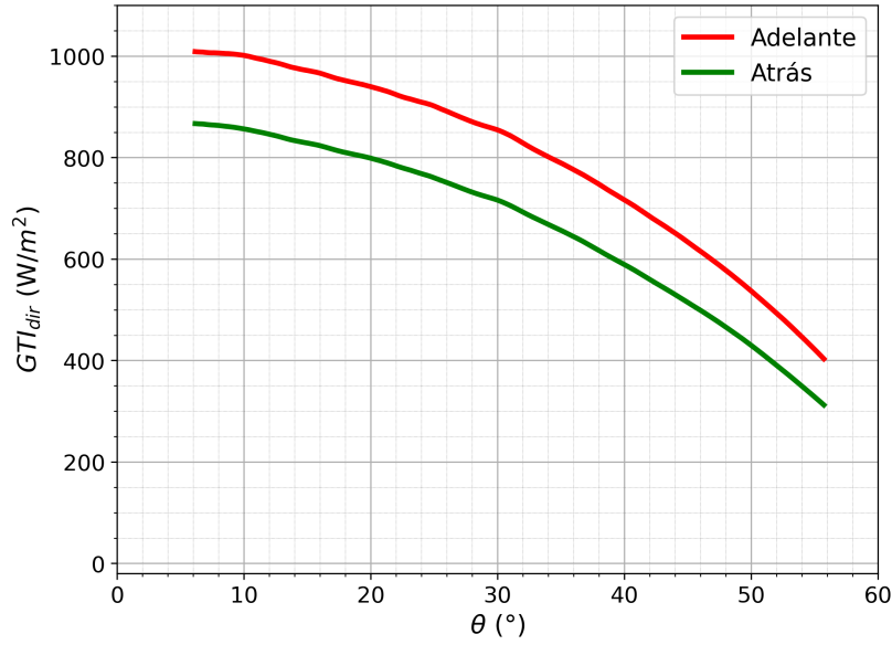
Figura 3.5: Estimación de irradiancia incidente desde la dirección del sol.
