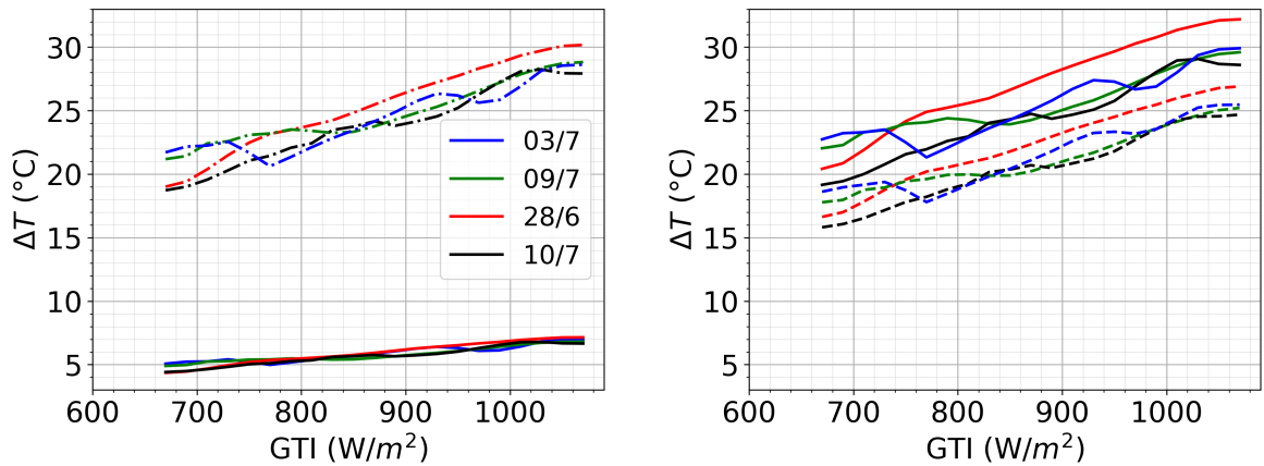
Figura 3.17: En el panel izquierdo se muestran: T_{out} - T_{in} (continua) y T_{al\ 2} - T_{in} (trazo-punto) para los 4 días contra la irradiancia. A la derecha se observan T_{al\ 3} - T_{in} (continua) y T_{al\ 1} - T_{in} (discontinua).
