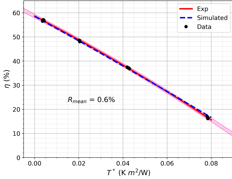
Figura 4.9: Curva de rendimiento del colector simulada comparada con la experimental.
