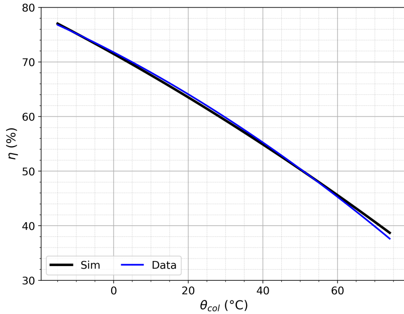
Figura 4.26: Comparación entre la curva simulada y el ensayo del SUN600.
