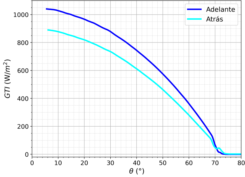
Figura 3.3: Medidas de irradiancia solar global en plano inclinado delante y detrás del vidrio.
