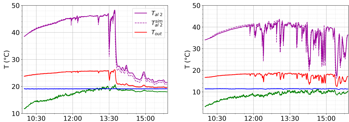
Figura 4.21: Temperatura a mitad de altura en el aluminio para el 3 de julio (izquierda) y el 9 de julio (derecha).
