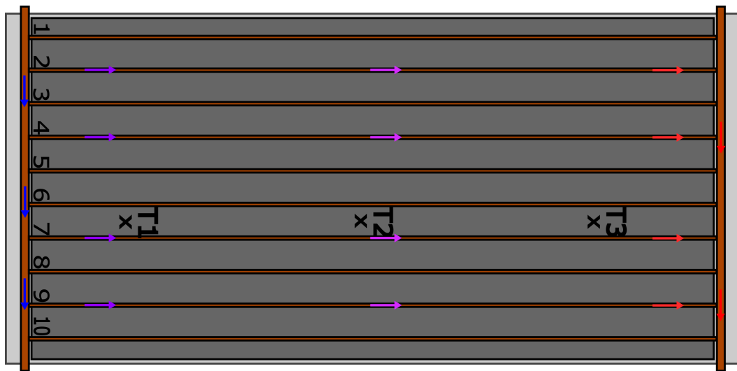
Figura 2.1: Esquema de la placa absorbedora y los tubos de cobre por los que circula agua.
