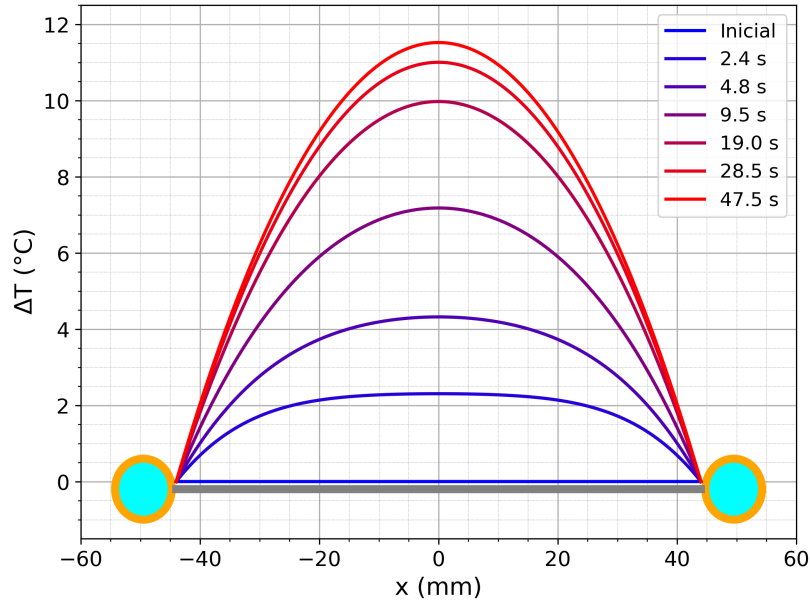
Figura 2.6: Ejemplo de incremento de la temperatura de la aleta con respecto a la inicial.
