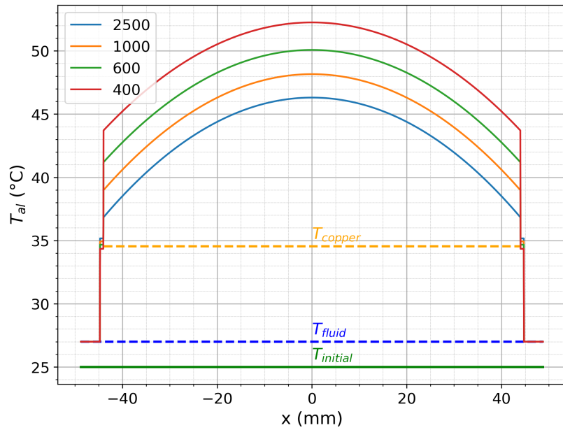
Figura 2.11: Perfil de temperaturas esperado de las aletas para distintos valores de h_{\text{cont}} en \text{W}/\text{m}^2\text{K} .
