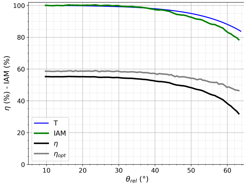
Figura 3.11: Cantidades adimensionales.
