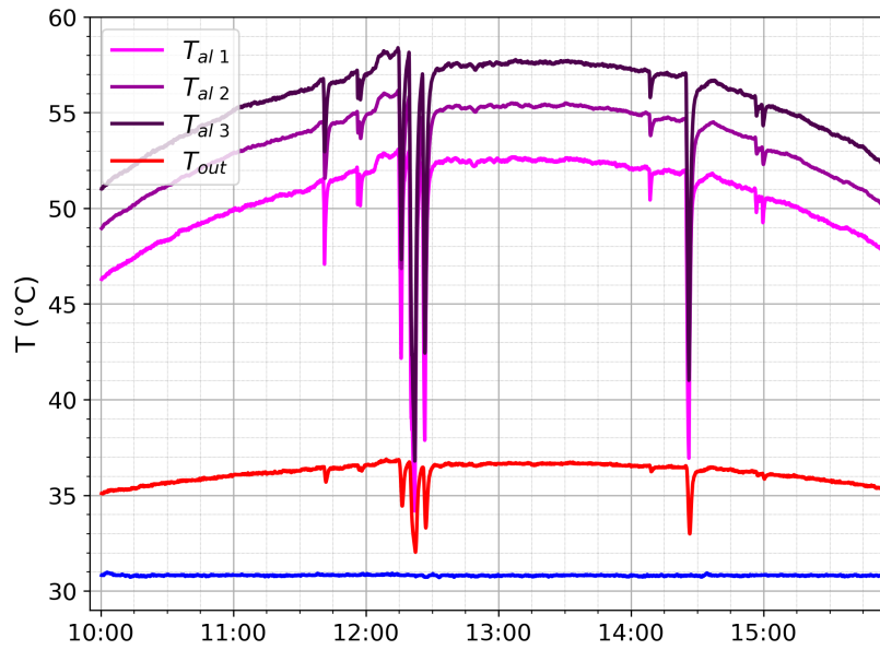
Figura 3.9: Medidas experimentales de temperatura de aluminio en 3 puntos del colector.
