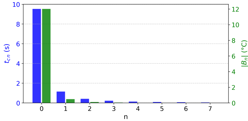
Figura 2.7: Serie de |B_n| y t_{cn} resuelta por Fourier.
