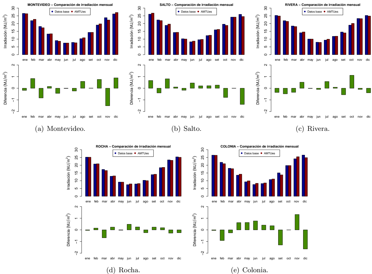
Figura 39: Comparación a escala mensual de los valores de irradiación GHI del AMTUes y los datos base.
