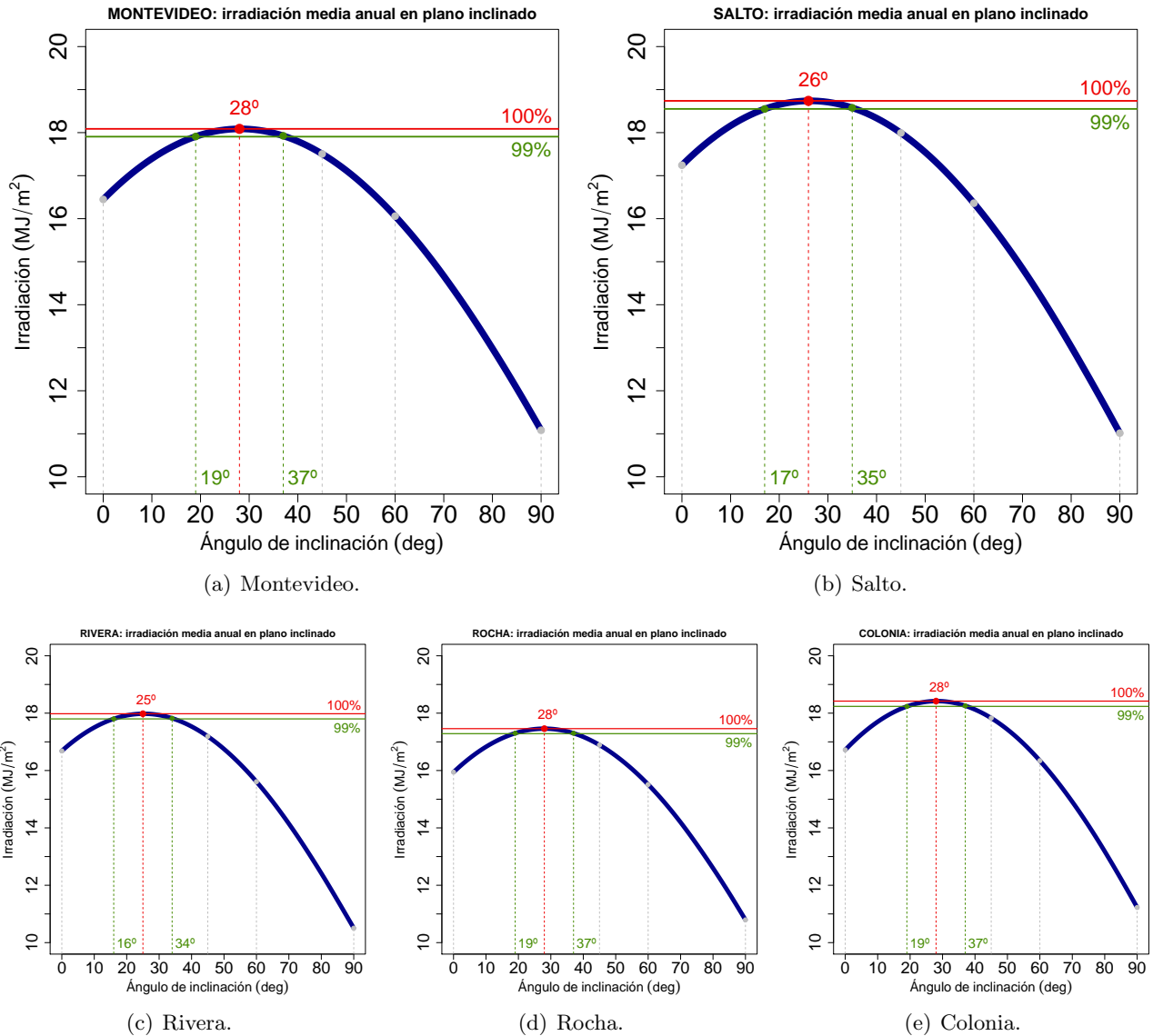
Figura 41: Variación de la irradiación anual con el ángulo de inclinación de las superficies de captación con orientación Norte. Se agrandan las imágenes de Montevideo y Salto como comparación Norte-Sur.
