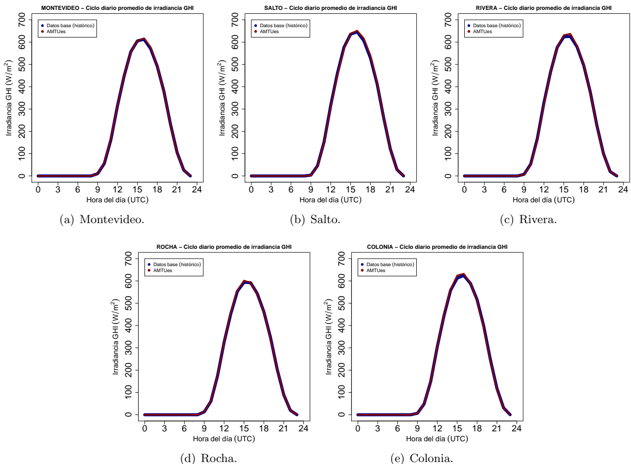
Figura 38: Ciclos diarios promedio de irradiancia solar para el AMTUes y los datos base.
