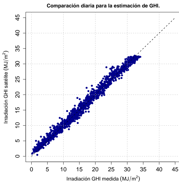
(a) Comparación de GHI.
