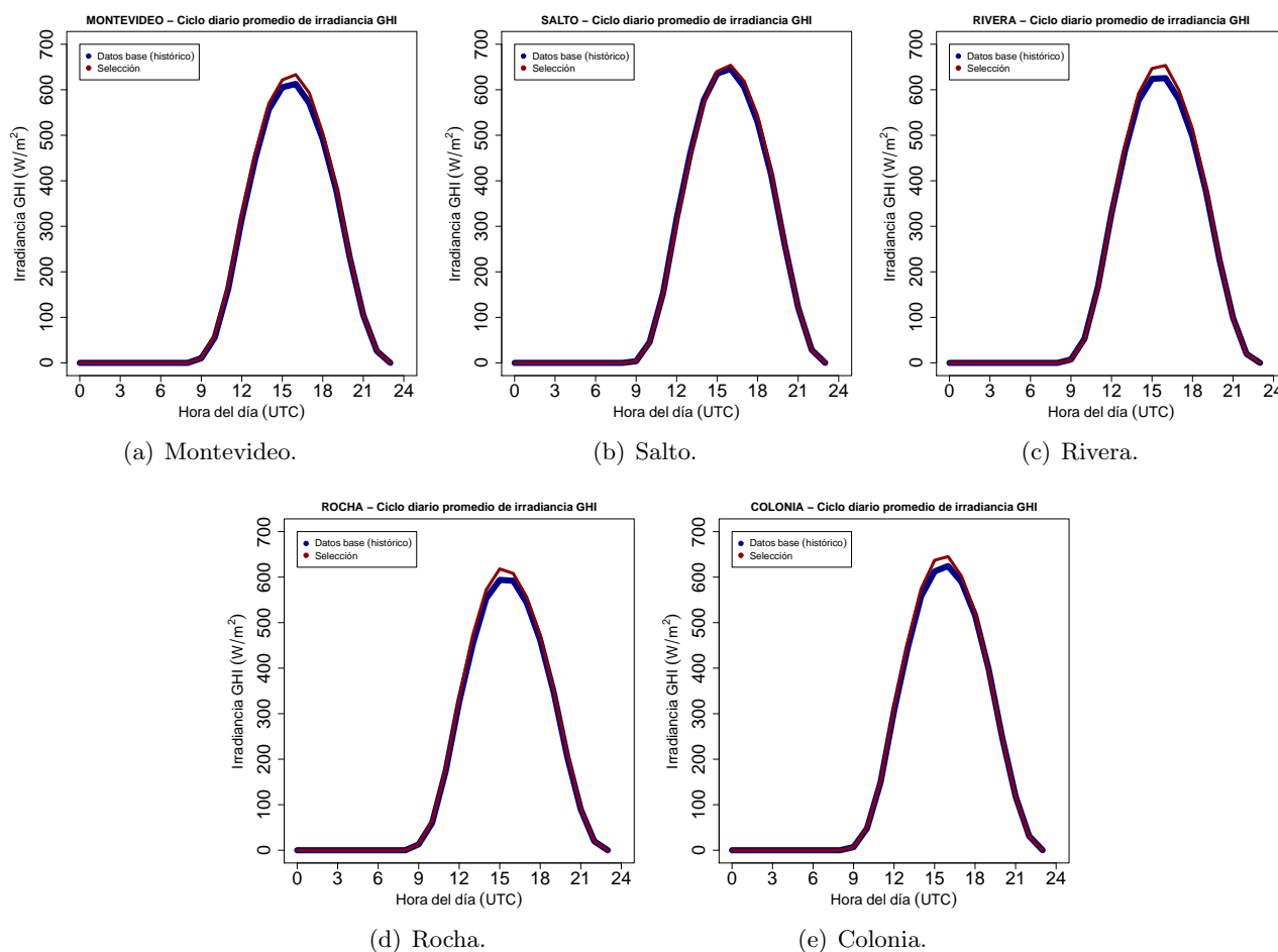
Figura 35: Ciclos diarios promedio de irradiancia solar para los meses seleccionados y los datos base. En la Sección 6.5 y en el Apéndice C se presentan gráficos iguales pero con los valores definitivos del AMTUs.
