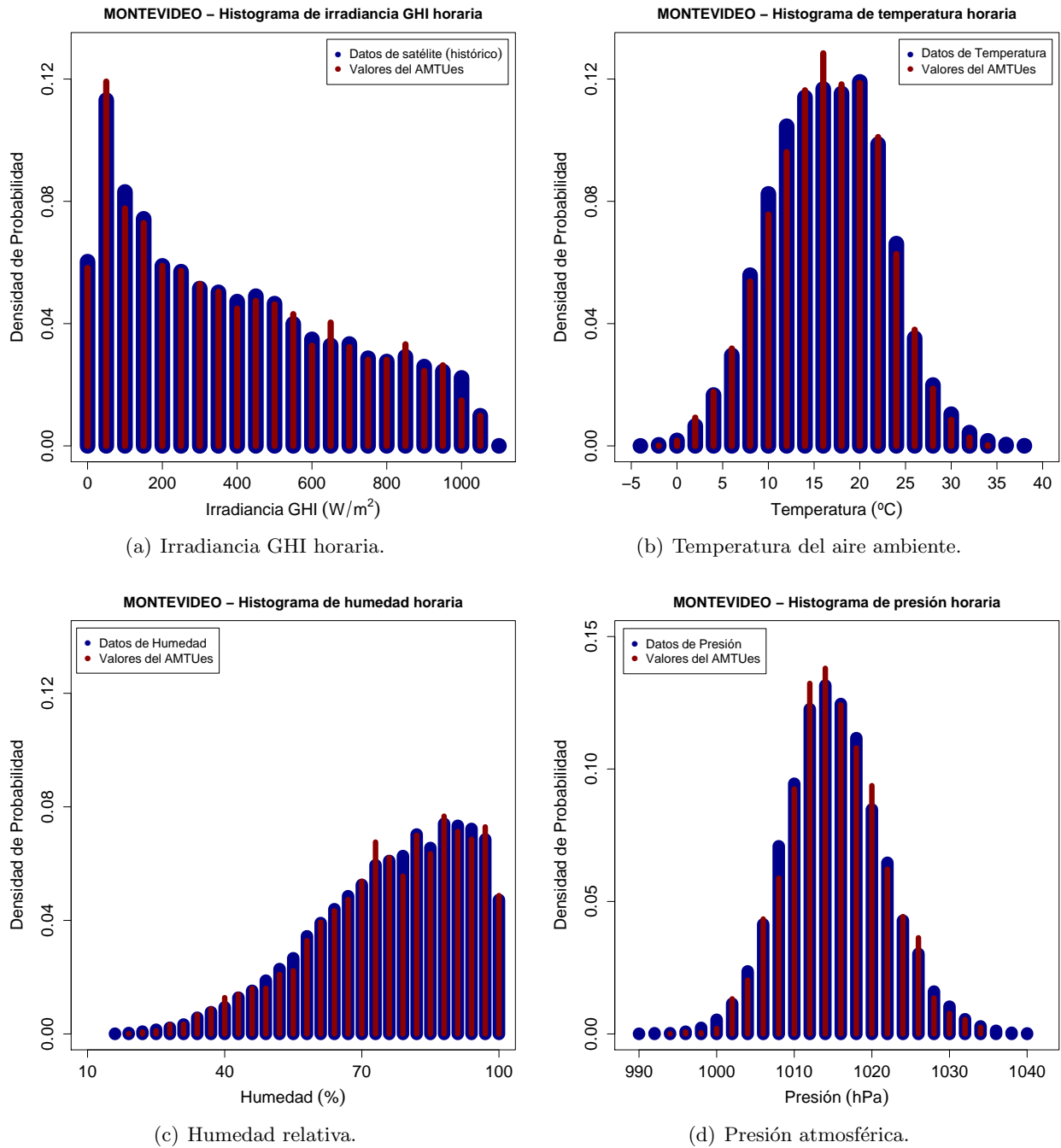
Figura 46: Comparación de los histogramas de los datos (horarios) del AMTUES de Montevideo contra los datos de largo plazo de la estación.
