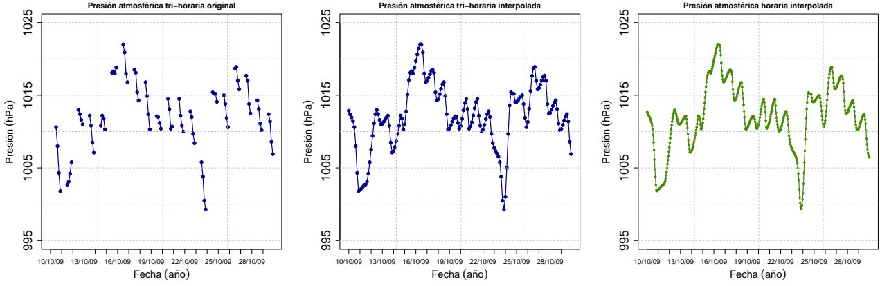
(a) Presión atmosférica tri-horaria original. (b) Presión atmosférica tri-horaria interpolada. (c) Presión atmosférica horaria interpolada.
