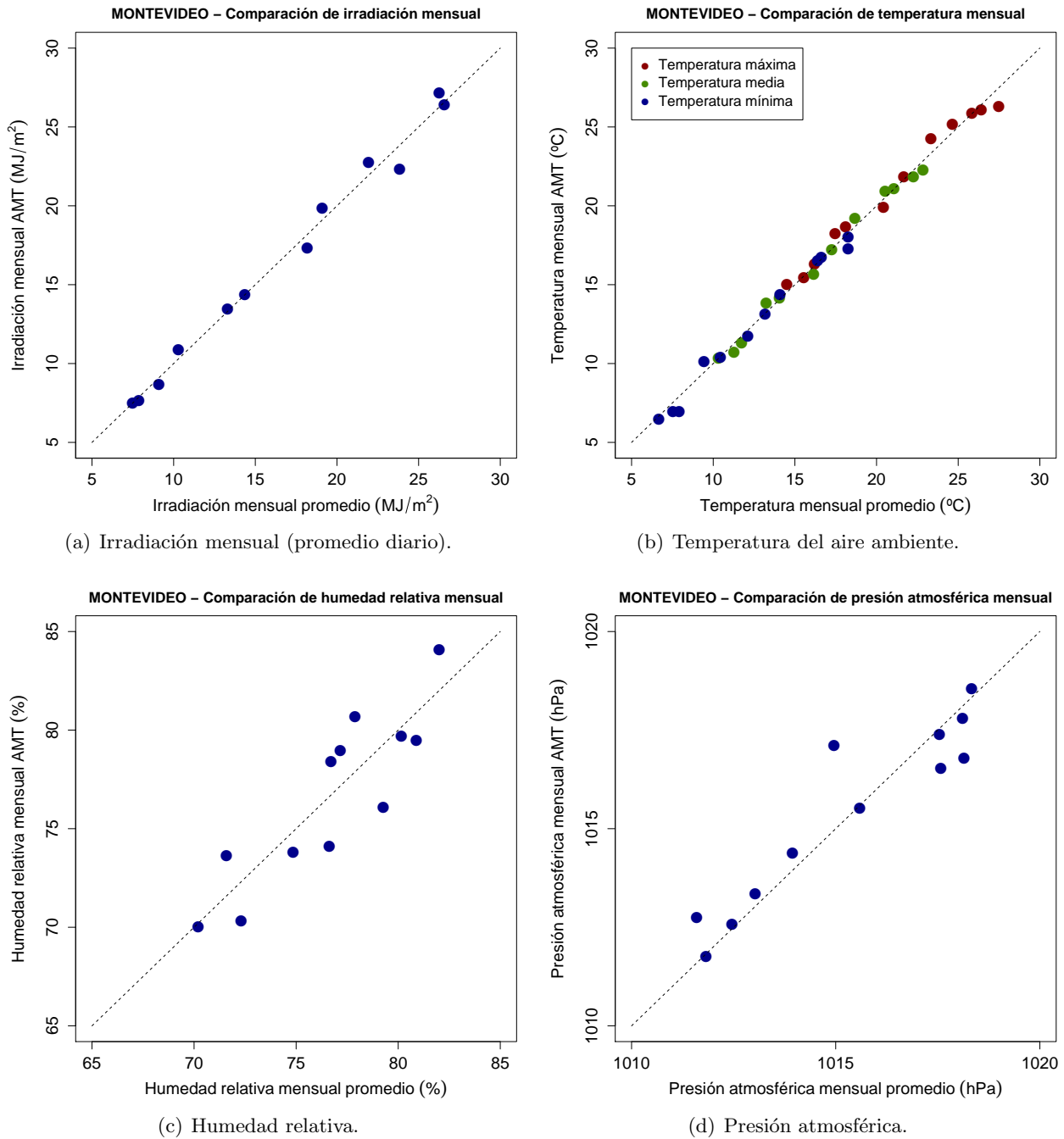
Figura 44: Comparación a escala mensual de los datos del AMT con las medias mensuales de los 15,0 años de datos para Montevideo.
