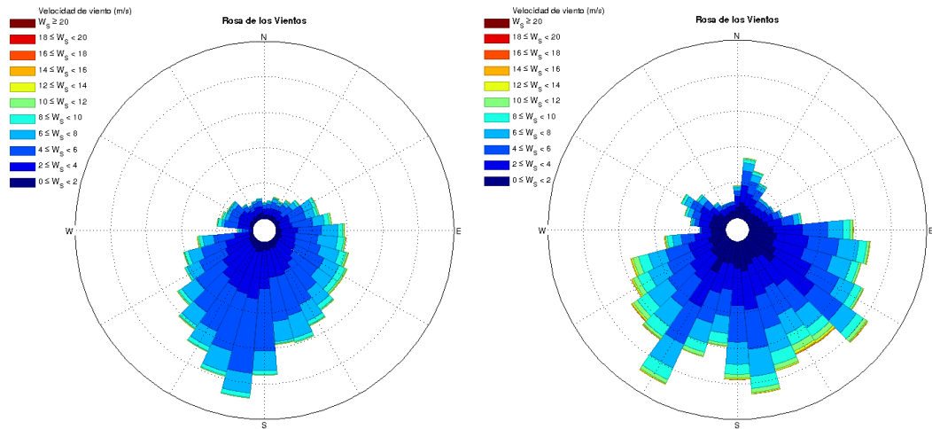
(a) Estación CR UTE (transportada a 20 m). Medida horaria. (b) Estación SS INIA (2 m). Medida horaria.
