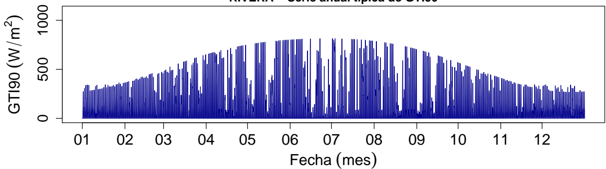
RIVERA – Serie anual típica de GTI90
