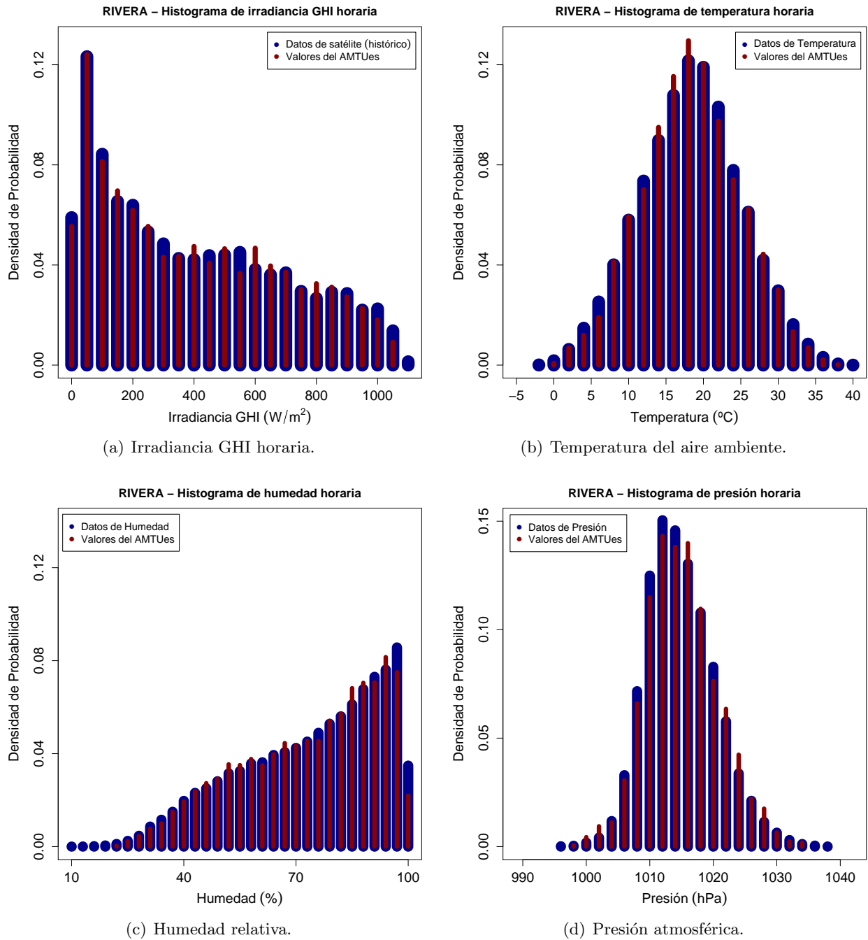
Figura 54: Comparación de los histogramas de los datos (horarios) del AMTUES de Rivera contra los datos de largo plazo de la estación.
