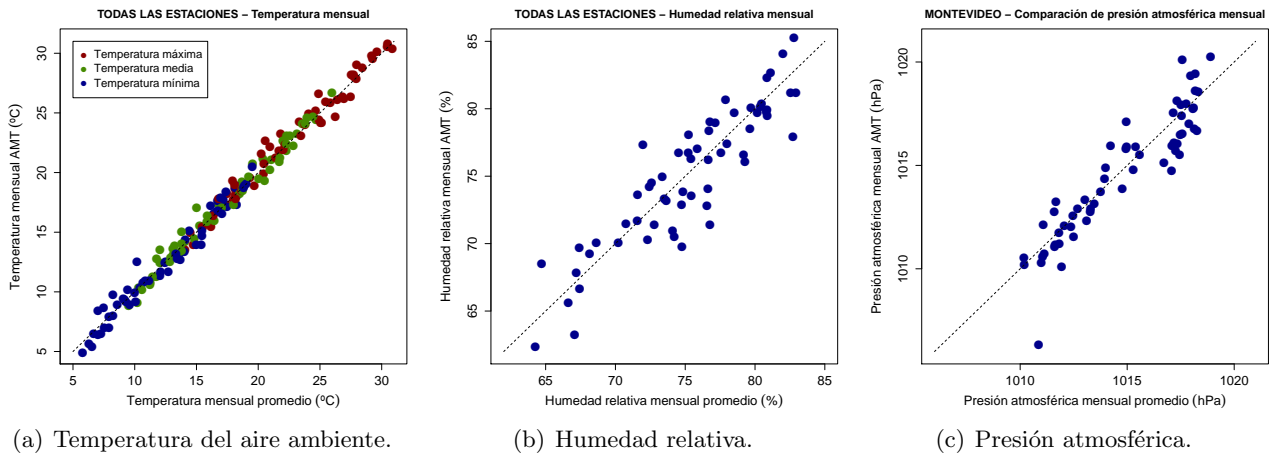
Figura 40: Comparación a escala mensual de las variables complementarias del AMTUES con las medias mensuales de los datos de largo plazo para las 5 localidades. El eje x se grafican las medias mensuales de los datos base y en el eje y las medias mensuales del AMTUES.
