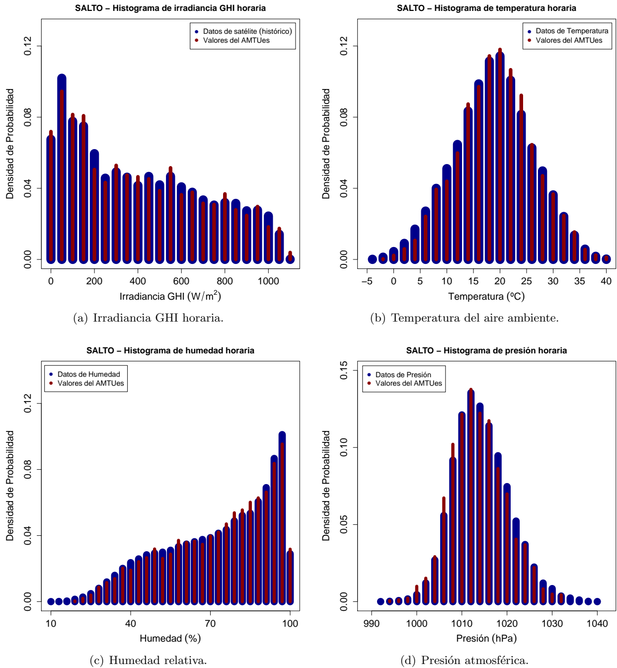
Figura 50: Comparación de los histogramas de los datos (horarios) del AMTUES de Salto contra los datos de largo plazo de la estación.
