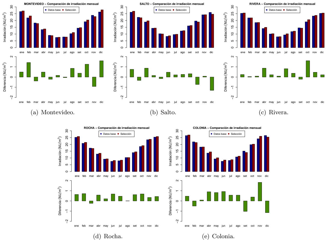
Figura 33: Comparación a escala mensual de los valores de irradiación GHI de los meses seleccionados y los datos de largo plazo. La comparación usando los datos del AMTUES se muestra en la Sección 6.5.
