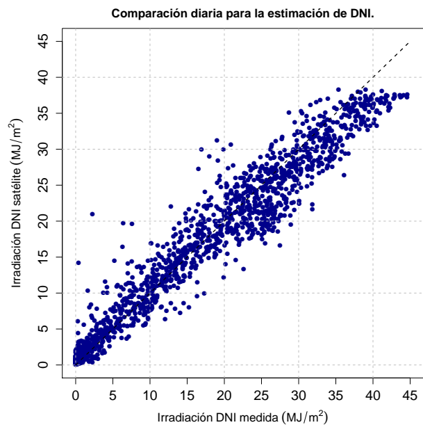
(b) Comparación de DNI.
