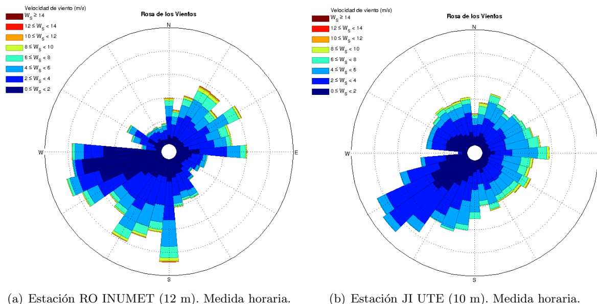
Figura 22: Rosa de los vientos para la localidad de Rocha. El ángulo es la dirección desde la cual proviene el viento.
