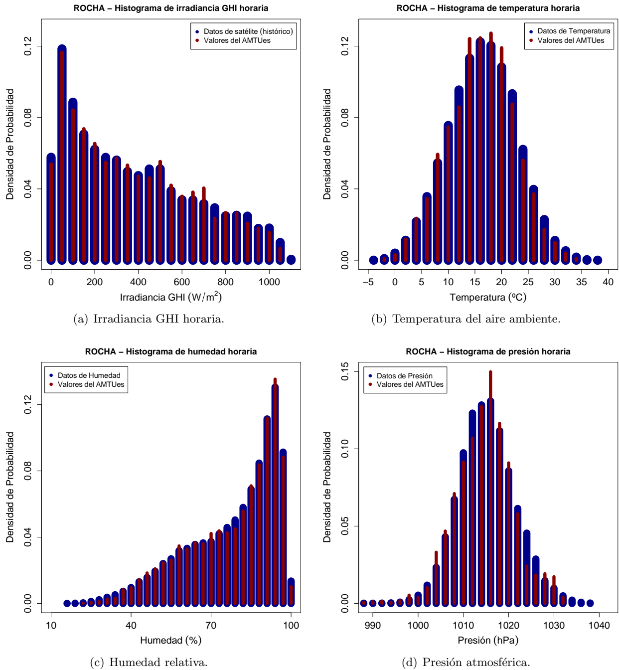
Figura 58: Comparación de los histogramas de los datos (horarios) del AMTUES de Rocha contra los datos de largo plazo de la estación.
